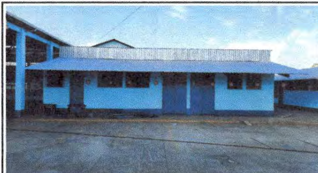
Foto 8: Sustrucción de lámina, por lámina troquelada aluzinc calibre 26 en módulo 4
